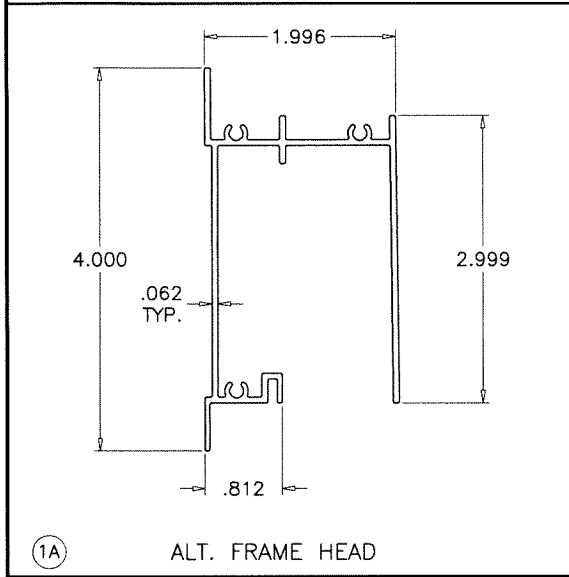
① FRAME HEAD/FRAME SILL TYPE '2'
